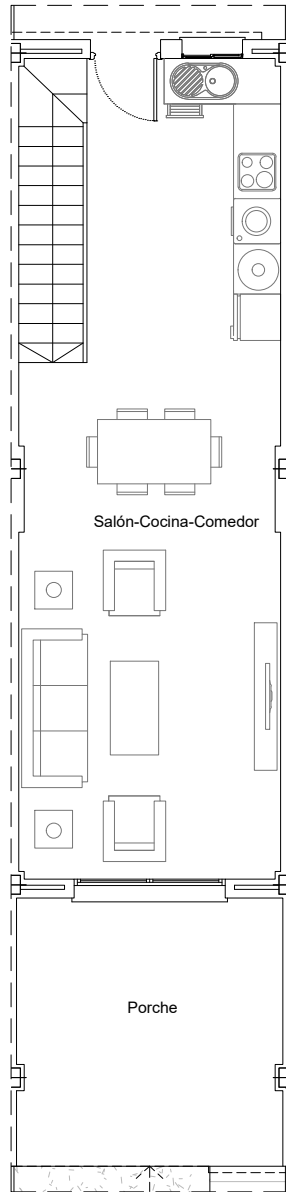
Planta Baja. 1:100
