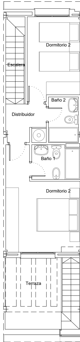
Planta Primera. 1:100
